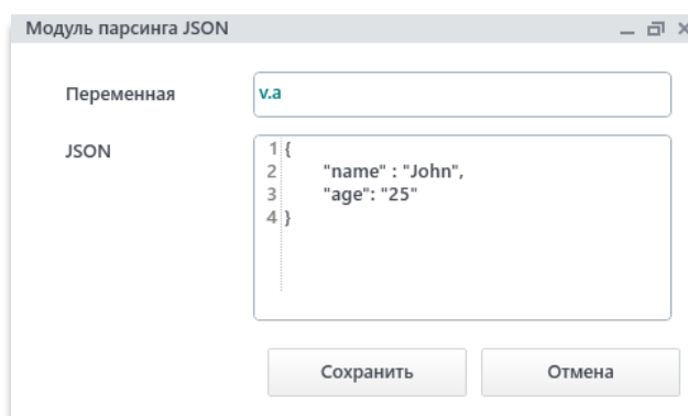
Рис. 12.44.2. Пример заполнения
