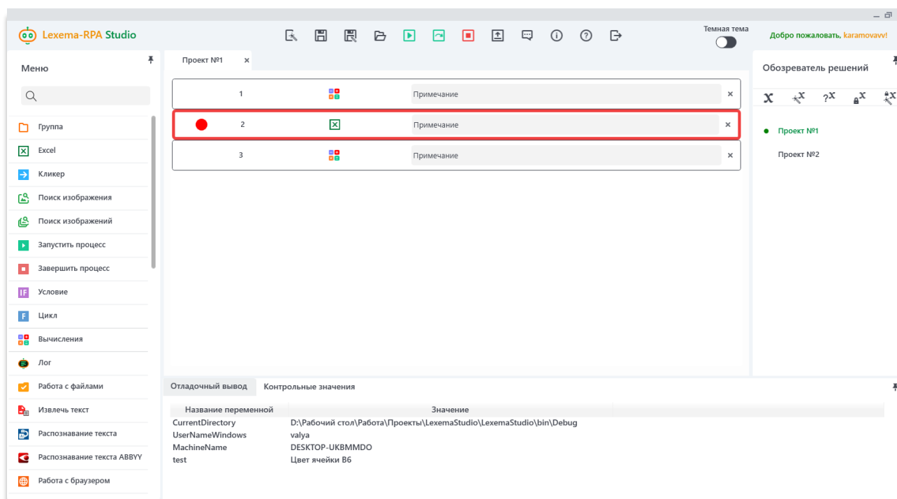
Рис. 1.2.12. Пошаговая отладка
