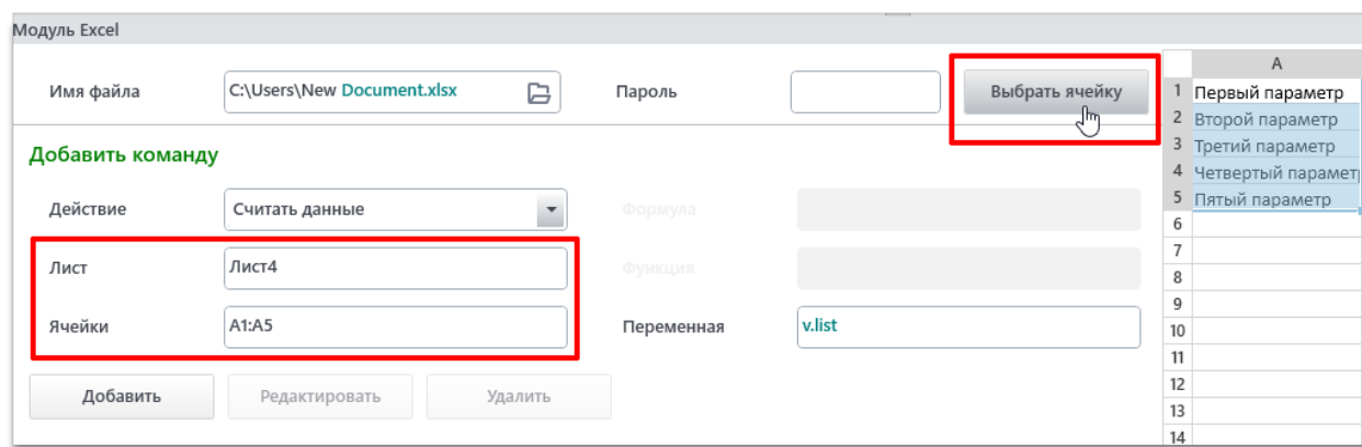
Рис. 2.3.9. Выбрать ячейку
