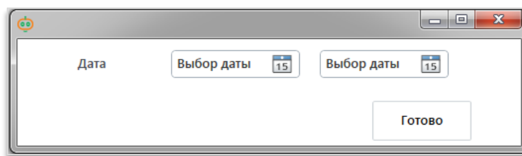
Рис. 9.30.3. Пример окна №2
