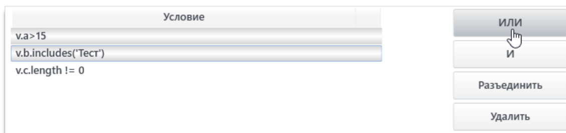
Рис. 6.16.4. Связывание условий
