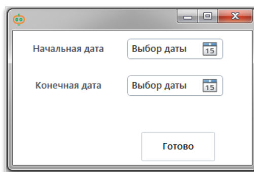
Рис. 9.30.2. Пример окна №1
