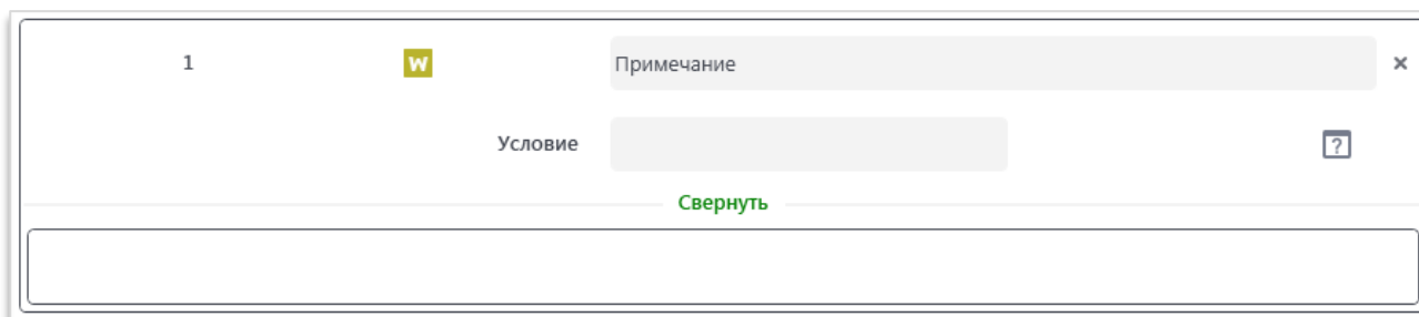
Рис. 6.21.1. Вид модуля
