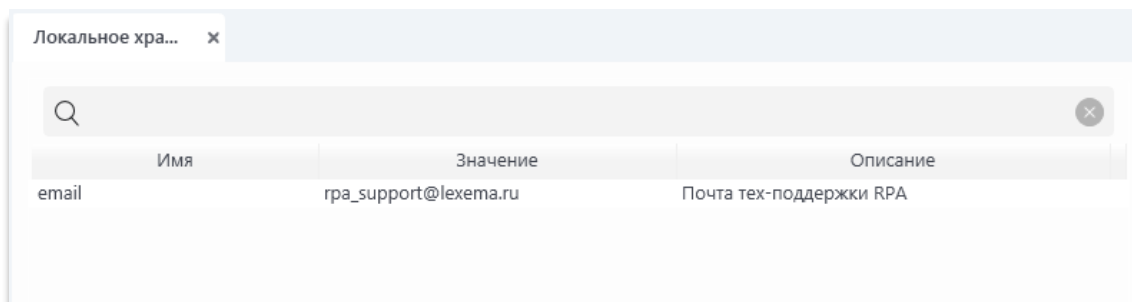
Рис. 1.1.16. Локальные переменные
