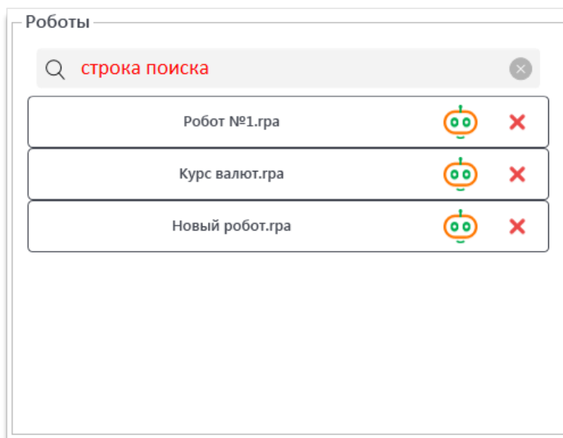
Рис. 13.54.1. Раздел «Роботы»
