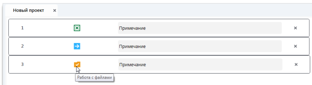
Рис. 1.2.9. Структура проекта
