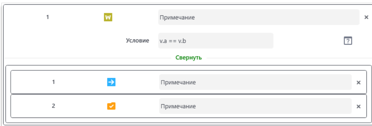
Рис. 6.21.2. Добавление действий
