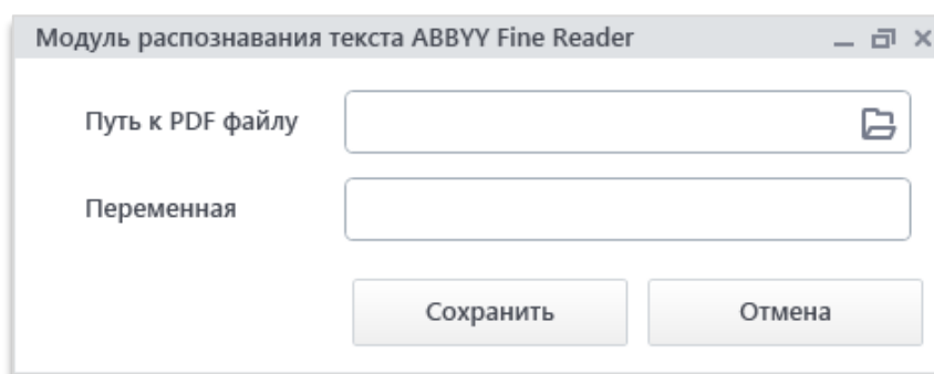
Рис. 10.34.1. Окно модуля
