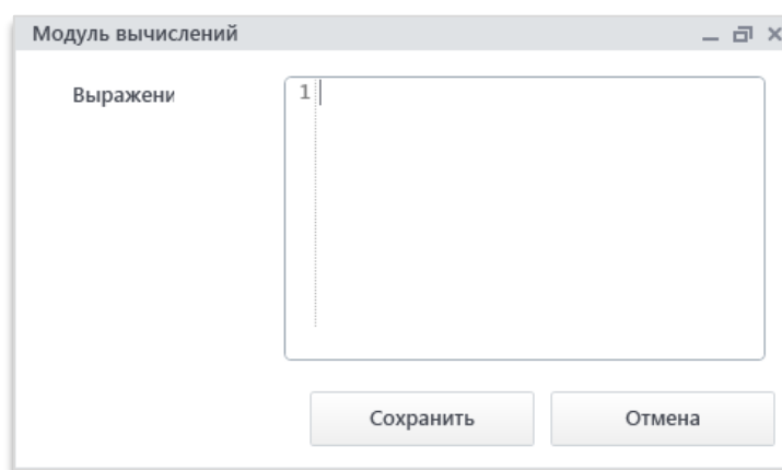
Рис. 12.37.1. Окно модуля
