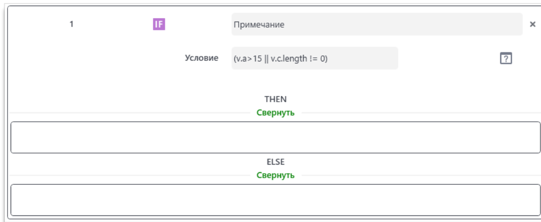
Рис. 6.16.9. Отображение условия
