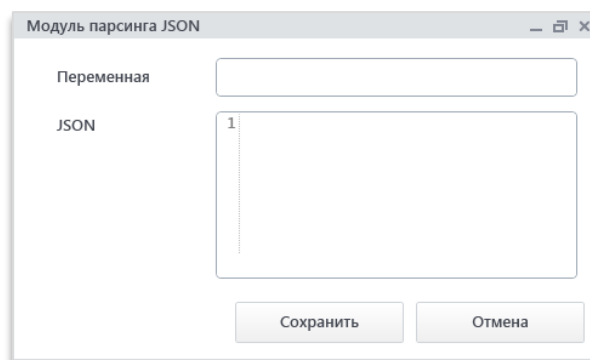
Рис. 12.44.1. Окно модуля
