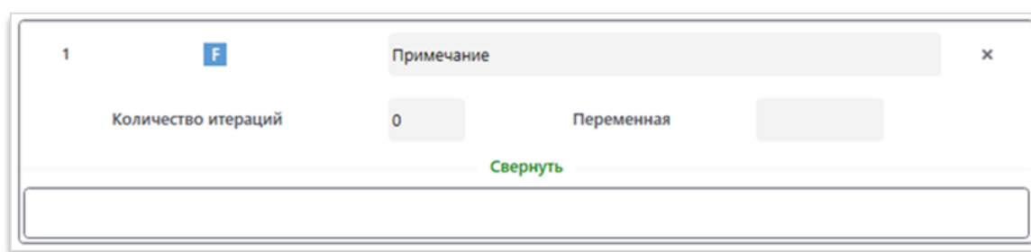
Рис. 6.17.1. Вид модуля
