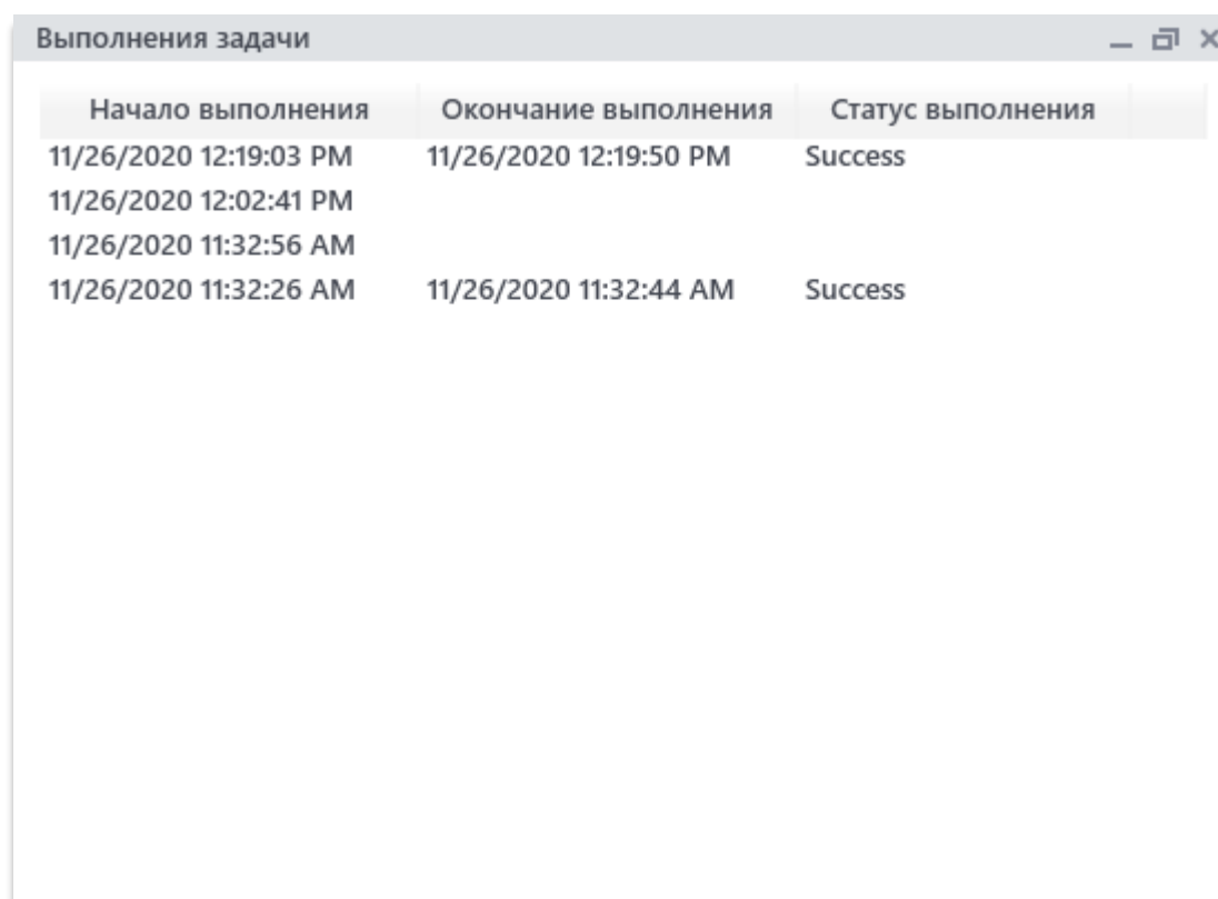
Рис. 13.55.2. Статистика выполнения
