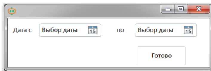
Рис. 9.30.4. Пример окна №3
