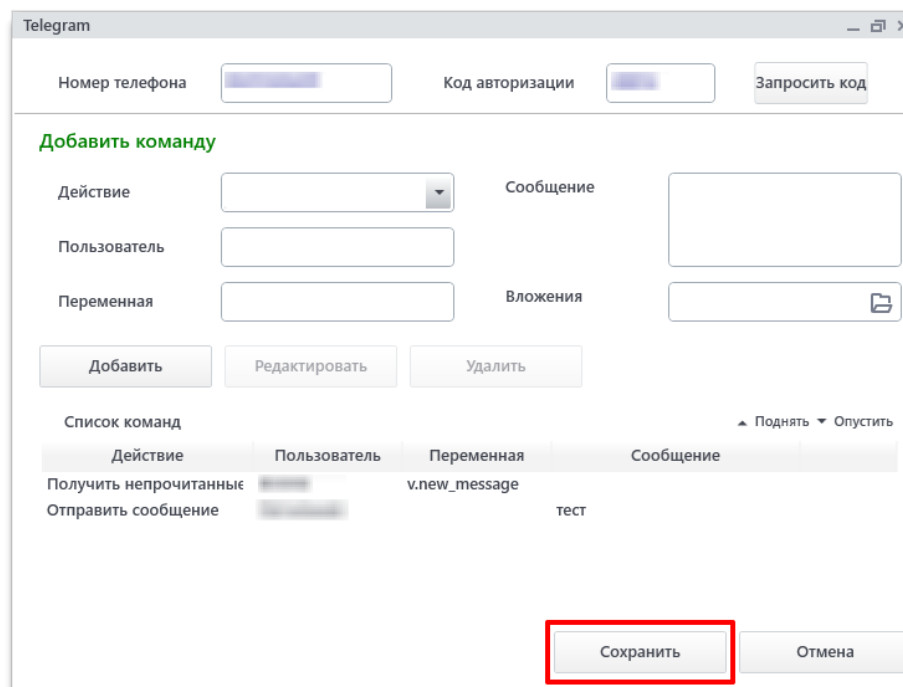
Рис. 11.35.3. Кнопка «Сохранить»
