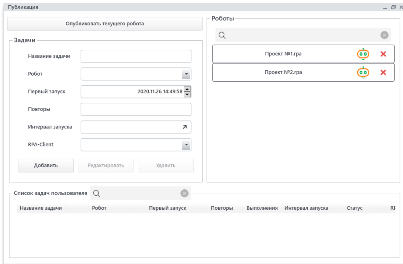
Рис. 13.52.1. Окно оркестратора
