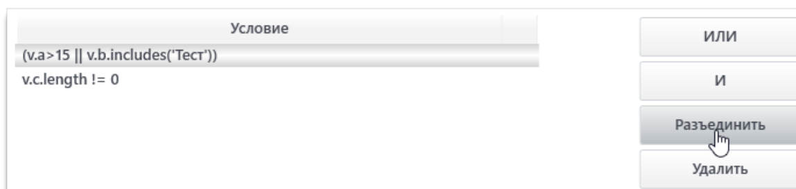
Рис. 6.16.6. Разъединение условий
