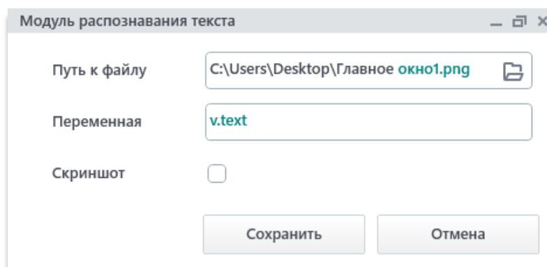
Рис. 10.33.1. Окно модуля
