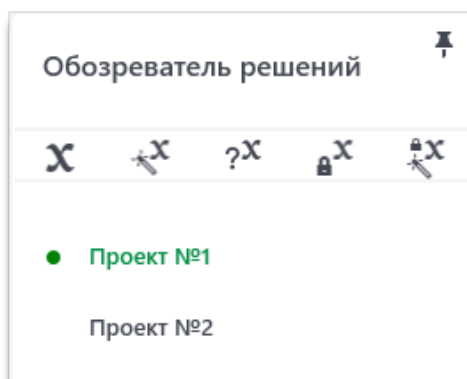
Рис. 1.1.13. Обзорщик решений
