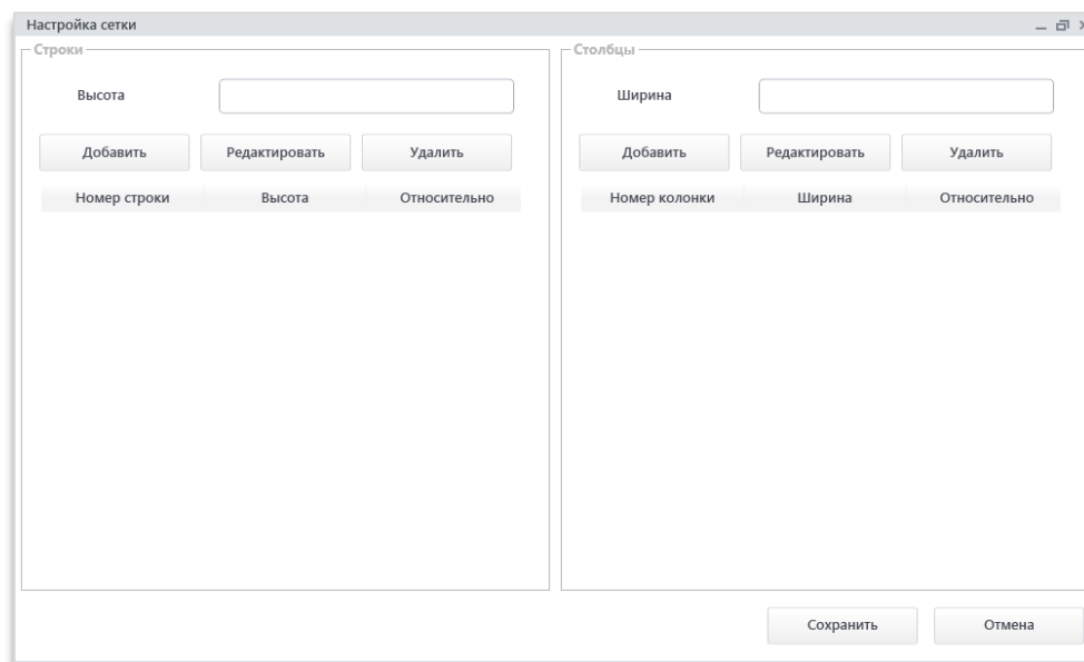
Рис. 9.30.1. Настройка сетки
