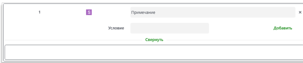
Рисунок 6.23.1. Модуль «Switch»
